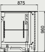
Banco basso refrigerato
